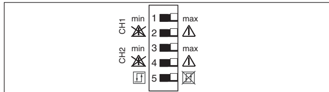
Рис. 3: DIL-переключатель VEGATOR 112
